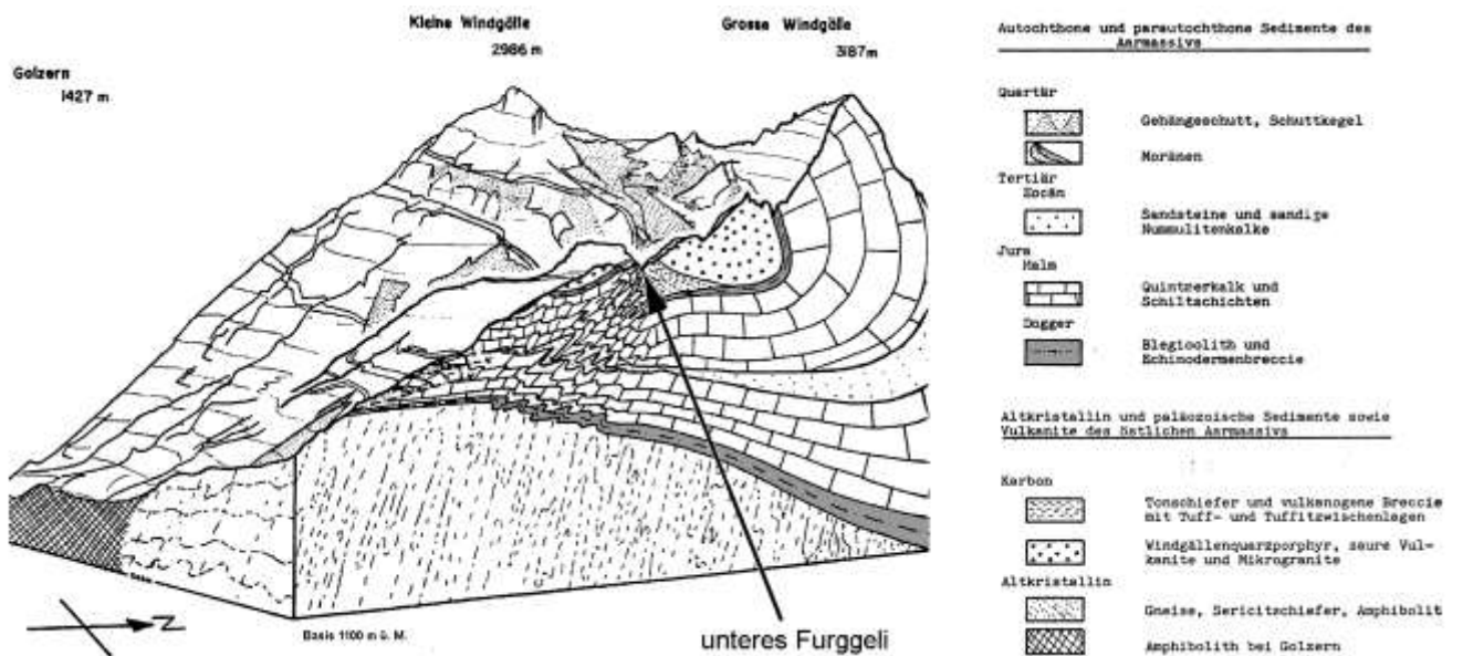
Profil aus: „Ergänzende Angaben zum Geologischen Rundgang“ (bei der Windgällenhütte) von Max Rothenfluh, Schattdorf
