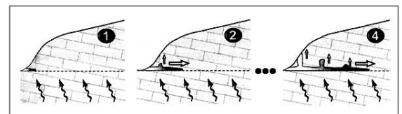
Abb. 7: Wasserspiegel Höhle
