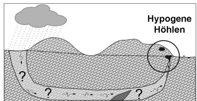
Abb. 2: hypogene Höhlen (Lukas Plan)
